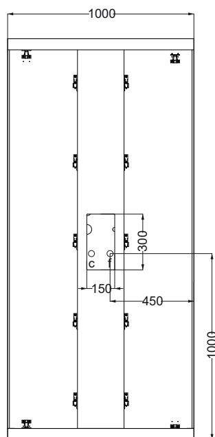
POSTERIORE
