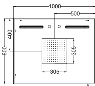
PIANTA
