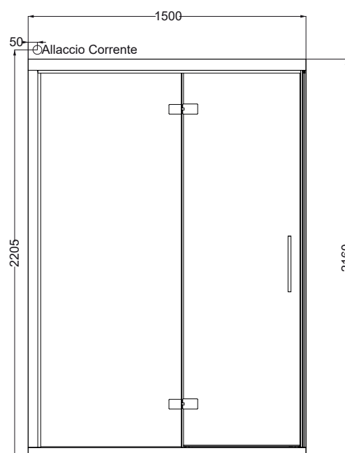
FRONTALE
